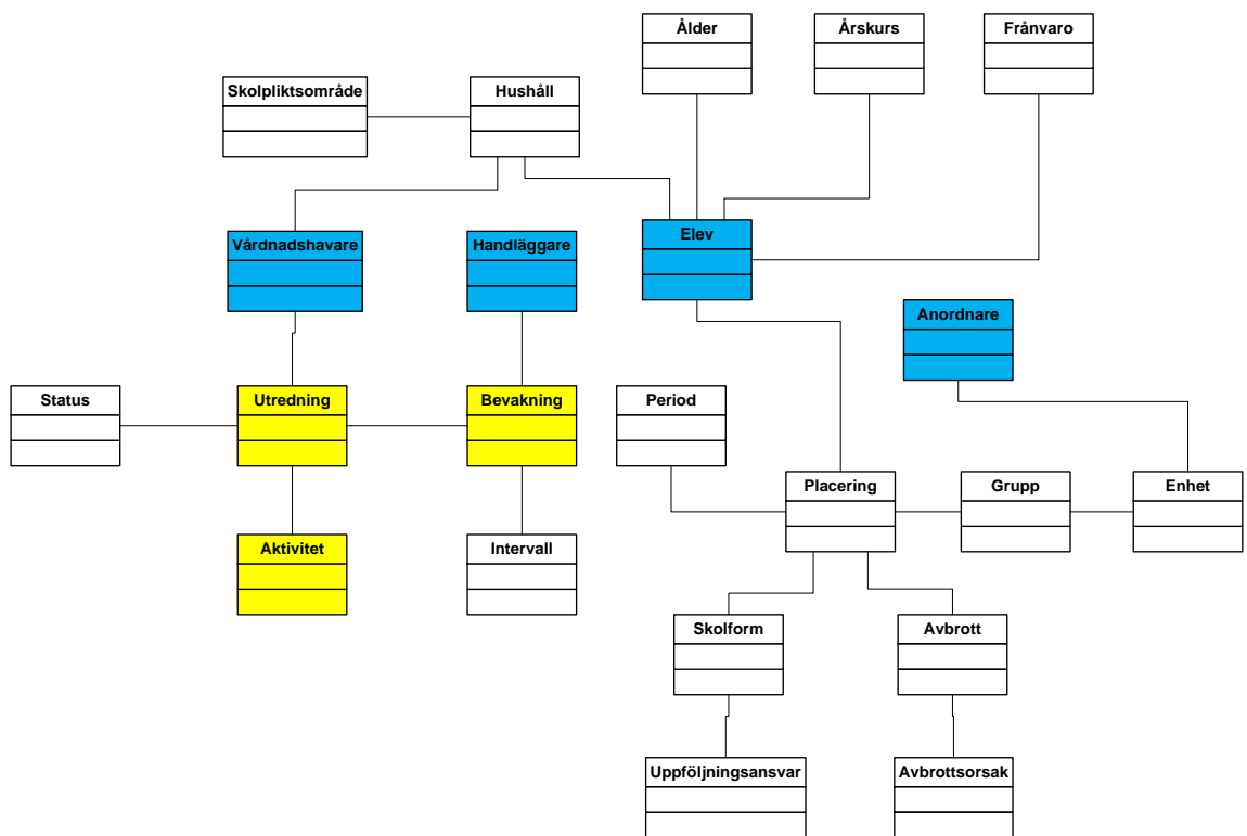
Figur 5. Informationsmodell skolplikt
