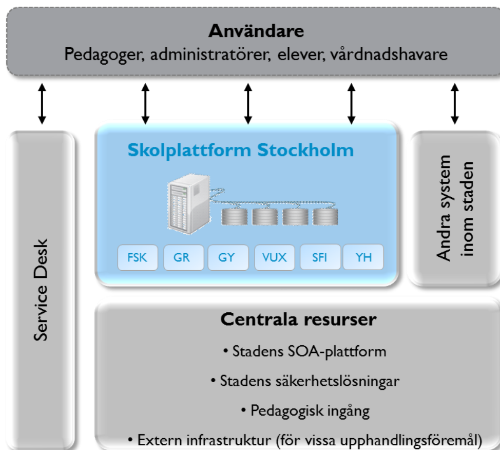
Figur 1 Konceptuell målbild för den framtida skolplattformen
